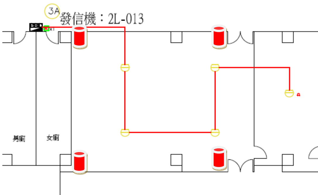
平面圖
